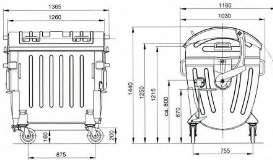
Схематичное изображение оцинкованного контейнера для мусора
